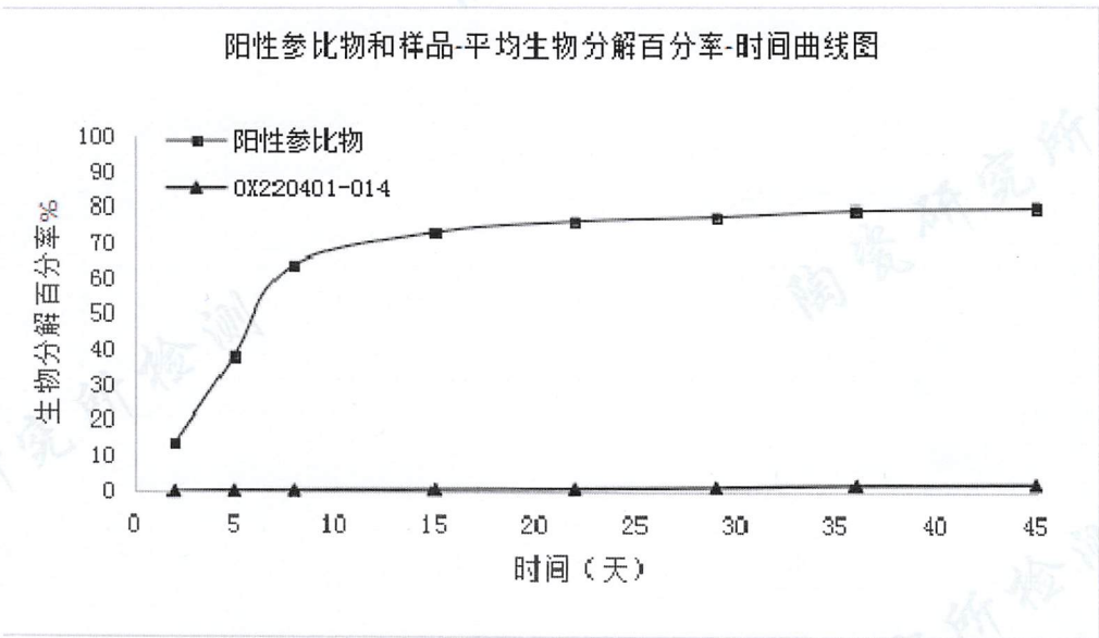
图 1.参比材料和样品组 (OX220401-014) 平均生物分解百分率-时间曲线图
